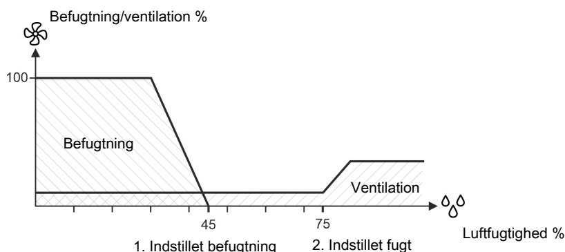
Figur 7: 1. Faldende luftfugtighed. Luftfugtigheden er under Indstillet befugtning. Staldcomputeren starter befugtningen. 2. Stigende luftfugtighed. Luftfugtigheden er over Indstillet fugt. Staldcomputeren øger ventilationen.
