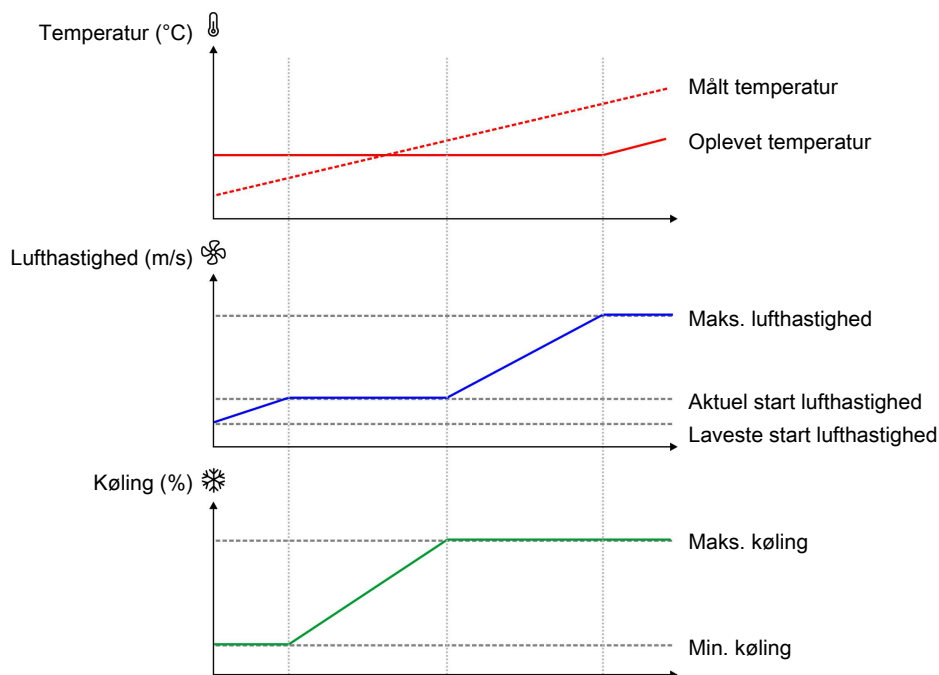
Figur 18: Kølingen starter allerede ved lav lufthastighed for at holde den ønskede indetemperatur. Når kølingen ikke kan holde temperaturen, øges lufthastigheden igen.
