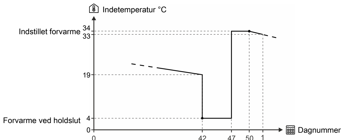
Figur 24: Eksempel på indstilling af forvarme.
