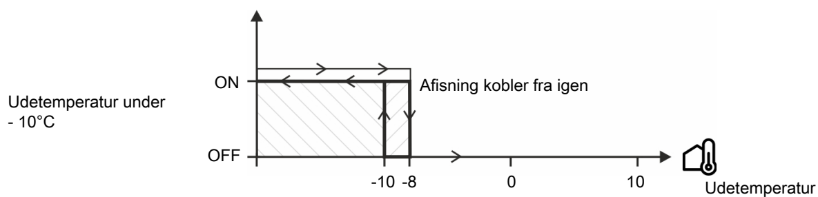
Figur 11: Aktivering af afisning
