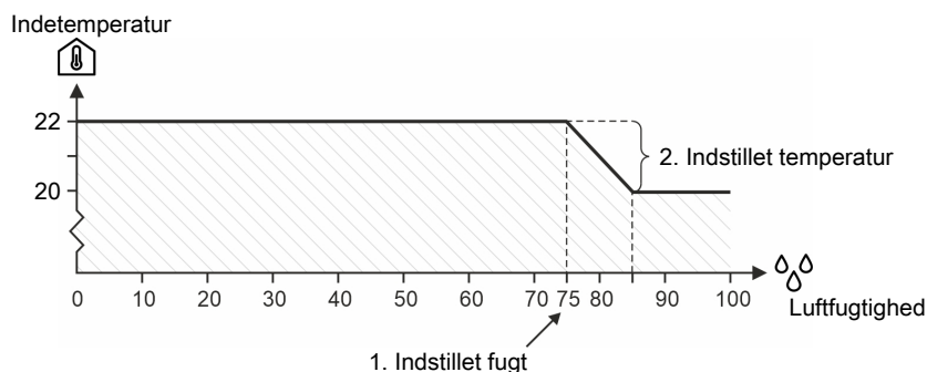
Figur 10: Fugtstyring med temperatursænkning
