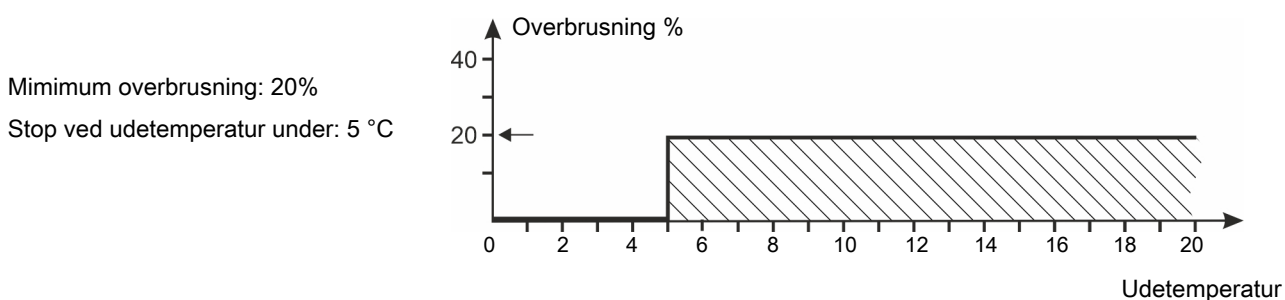
Figur 14: Overbrusning efter udetemperatur
