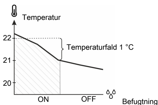
Figur 8: Faldende temperatur: Befugtningen vil blive afbrudt hvis indetemperaturen er 1 °C under Indstillet temperatur. Befugtningen vil ellers kunne få indetemperaturen til at falde yderligere.
