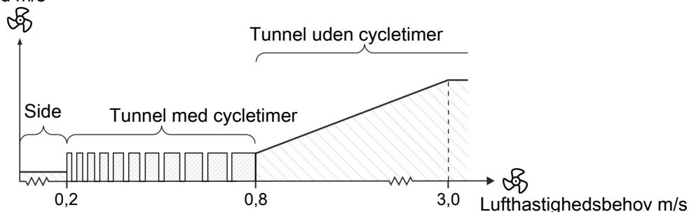
Figur 12: Ventilationsforløb med cycletimer ved tunnel-ventilation
