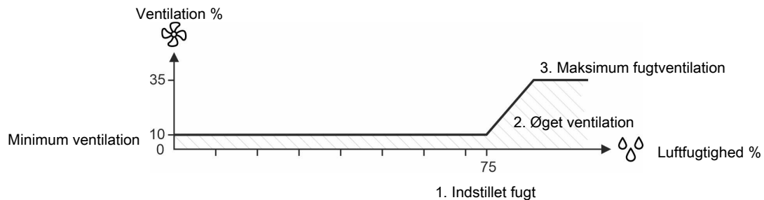
Figur 9: Fugtventilation: 1. Luftfugtigheden overstiger indstillet fugt. 2. Staldcomputeren øger ventilation. 3. Forøgelse op til maksimum fugtventilation (35 %).
